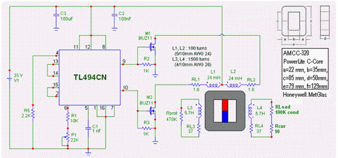
1. ábra. A kapcsolási rajz (Naudin 3. verziója)
